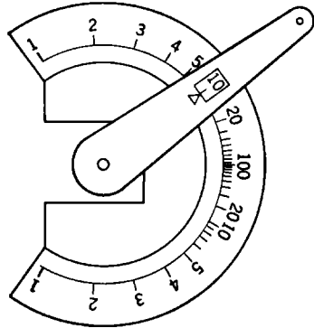
FIG. 3-4.—Output scale.
